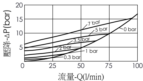
性能曲線
