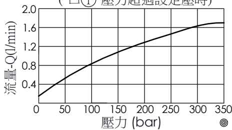
導壓流量 口①到口③ ("口①"壓力超過設定壓時)
