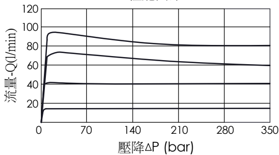
性能曲線
