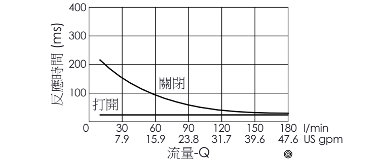
此曲線或數據僅供參考, 因為取決於客人使用的壓力、流量、液壓油黏度、清潔度、溫度等條件而有所不同
